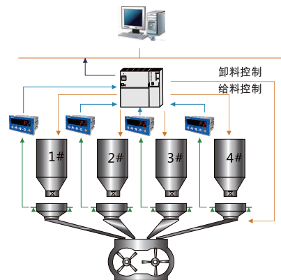
多物料并行配料称重应用
