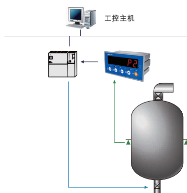
称重显示及重量数据传送应用
