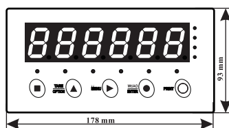
前面板尺寸(mm): 178×93
