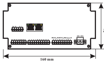
后面板尺寸(mm): 160×76
